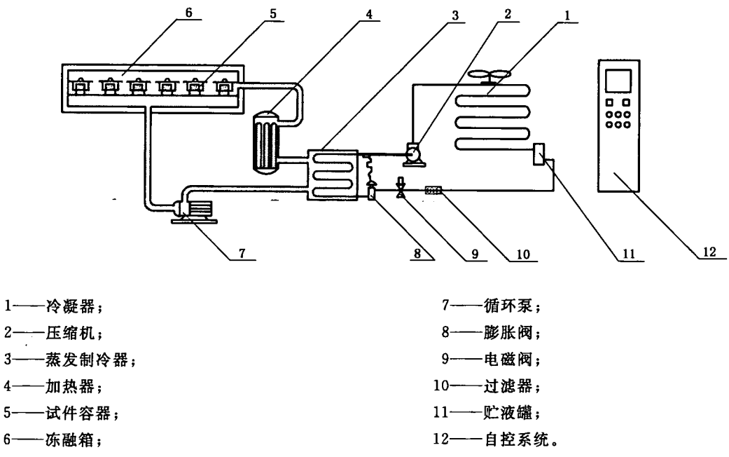
图 3 单边冻融试验设备系统示意图
