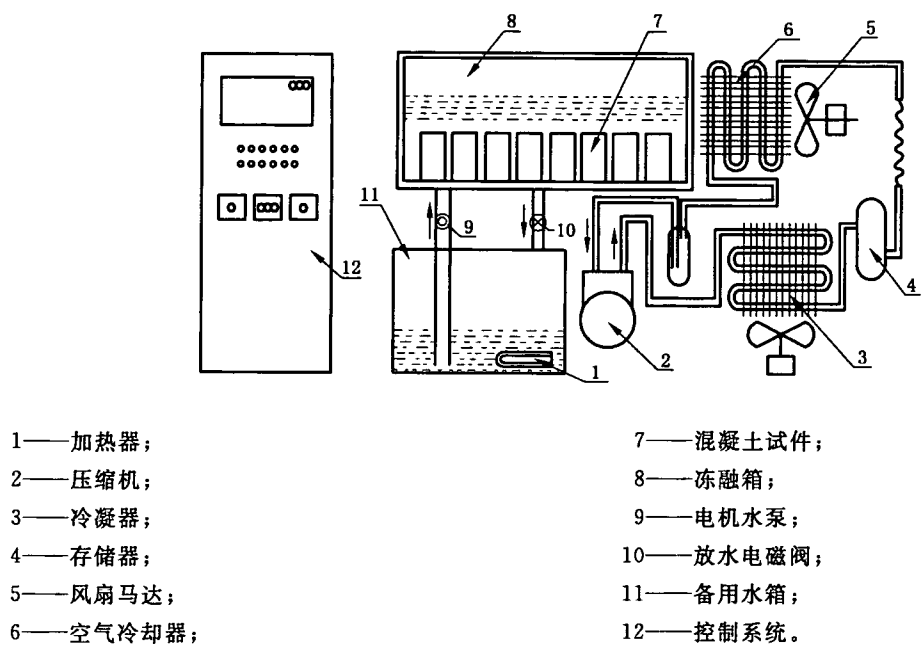
图 2 慢速冻融试验设备系统示意图
