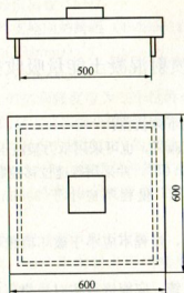
图 F.0.2 四边简支板的加载方式 (mm)
