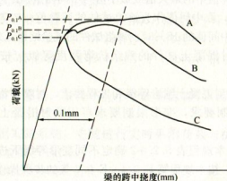
图 E.0.4 荷载-挠度曲线
