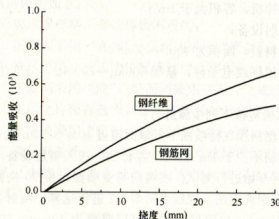
图 F.0.3-2 “能量-挠度”曲线
