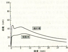
图 F.0.3-1 “荷载-挠度”曲线
