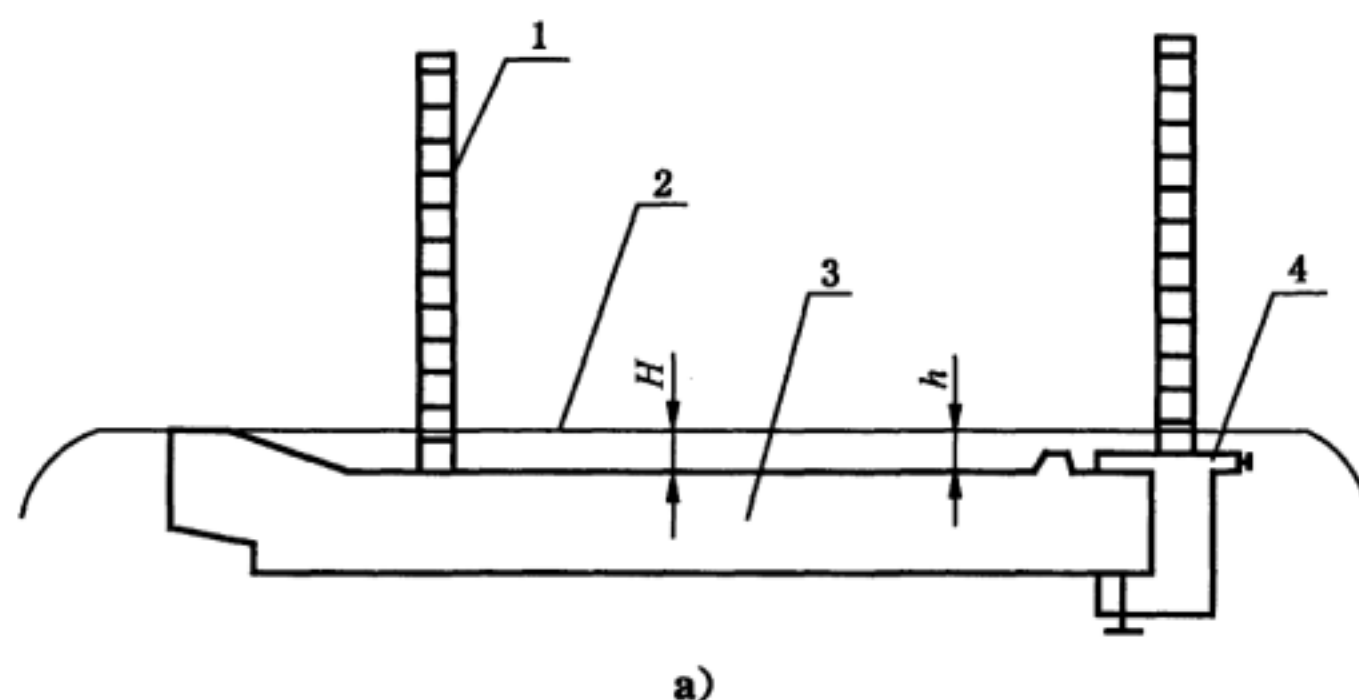
图 5 弯曲度测量位置示意图
