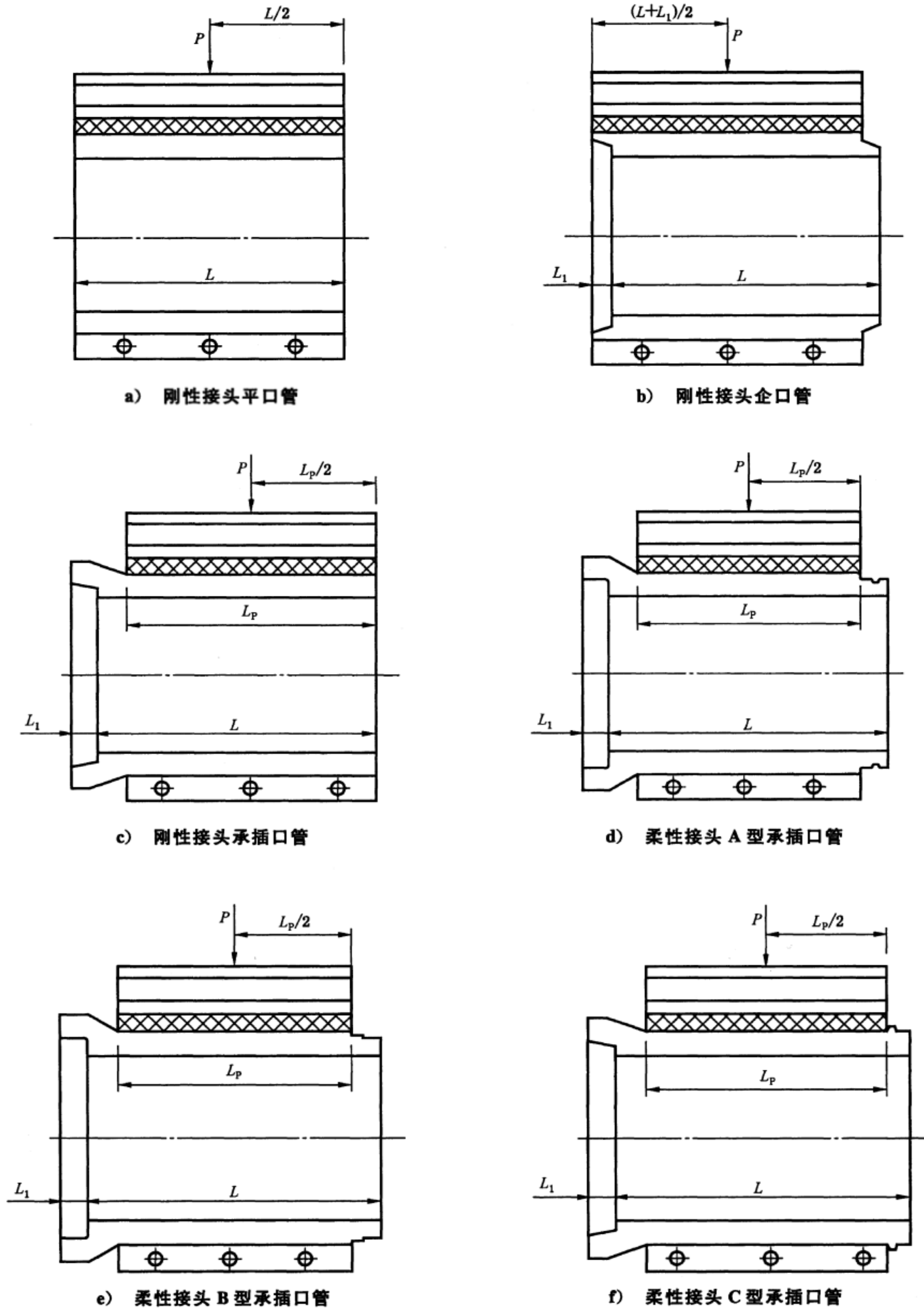
图 C.2 外压荷载试验装置加荷位置示意图
