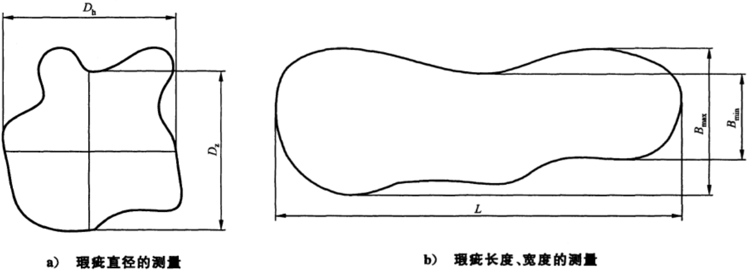
图 1 瑕疵尺寸测量示意图
