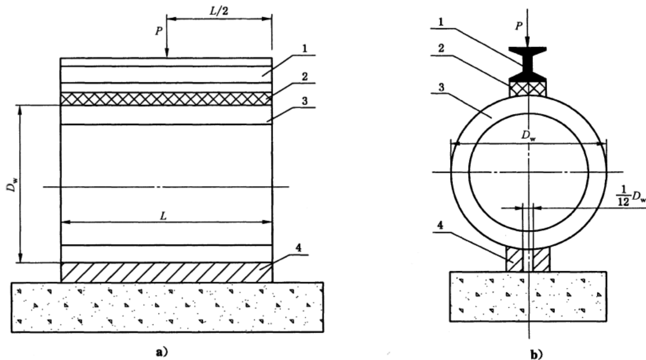
图 C.1 外压荷载试验装置示意图
