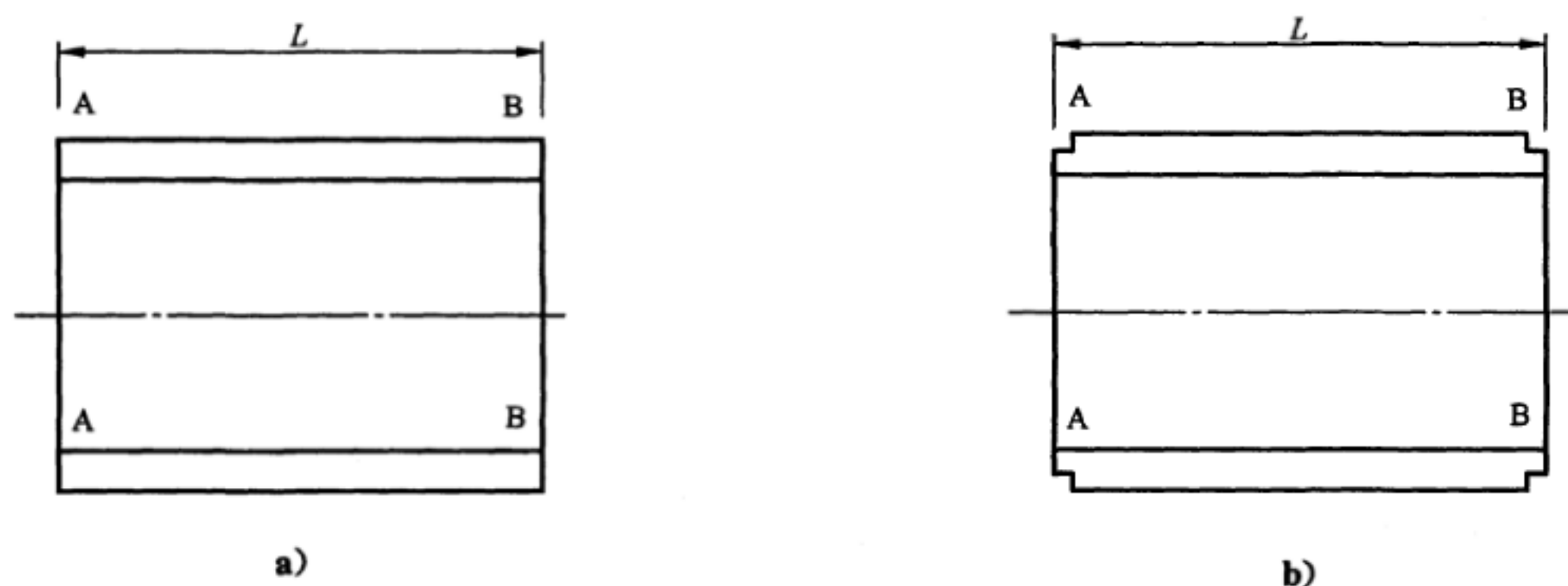
图 3 管体有效长度测量方法示意图
