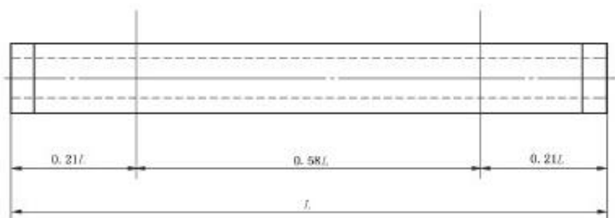
图4 两点吊吊点位置示意图
