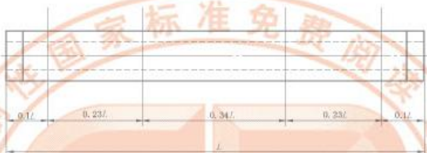
图5 四点吊吊点位置示意图
