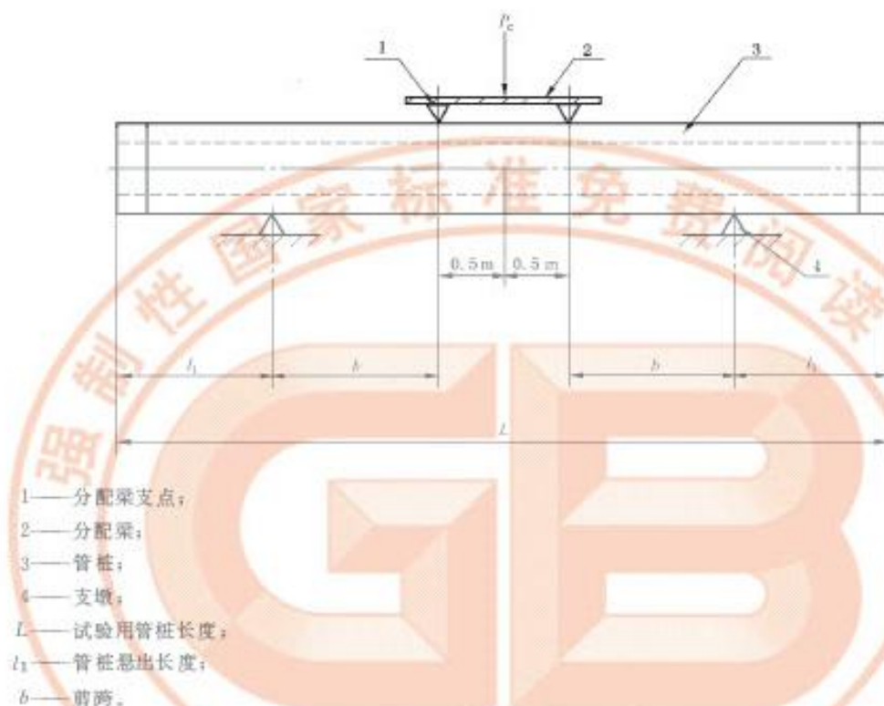
图 C.1 管桩抗剪试验示意图
