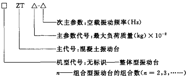
图1 振动台型号说明
