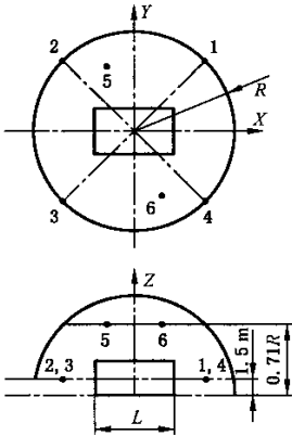
图 3 半球面上的传声器布置
