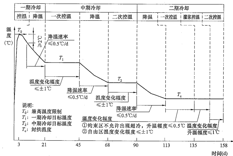
图1 溪洛渡拱坝混凝土温度控制示意图
