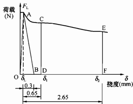
图 B.0.6 荷载-挠度简图
