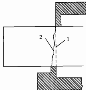
图 D.0.4 剪切破坏示意
