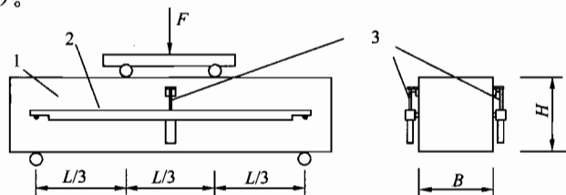
图 C.0.5 试验装置示意
