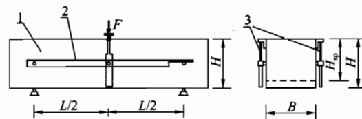
图 B.0.5 试验装置示意
