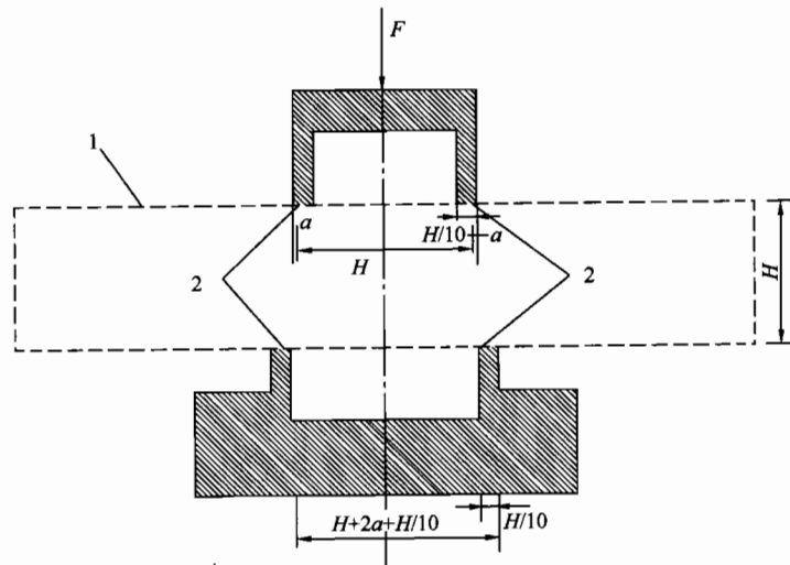
图 D.0.3 双面剪切试验装置简图
