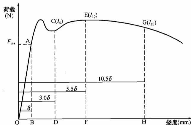
图 C.0.6 弯曲韧性指数定义示意
