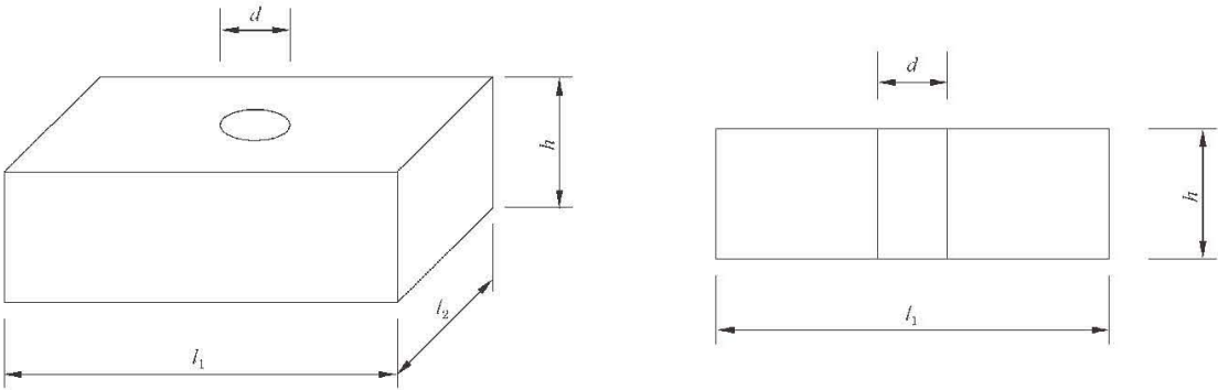
图 1 带竖孔内置箱体成孔芯模
