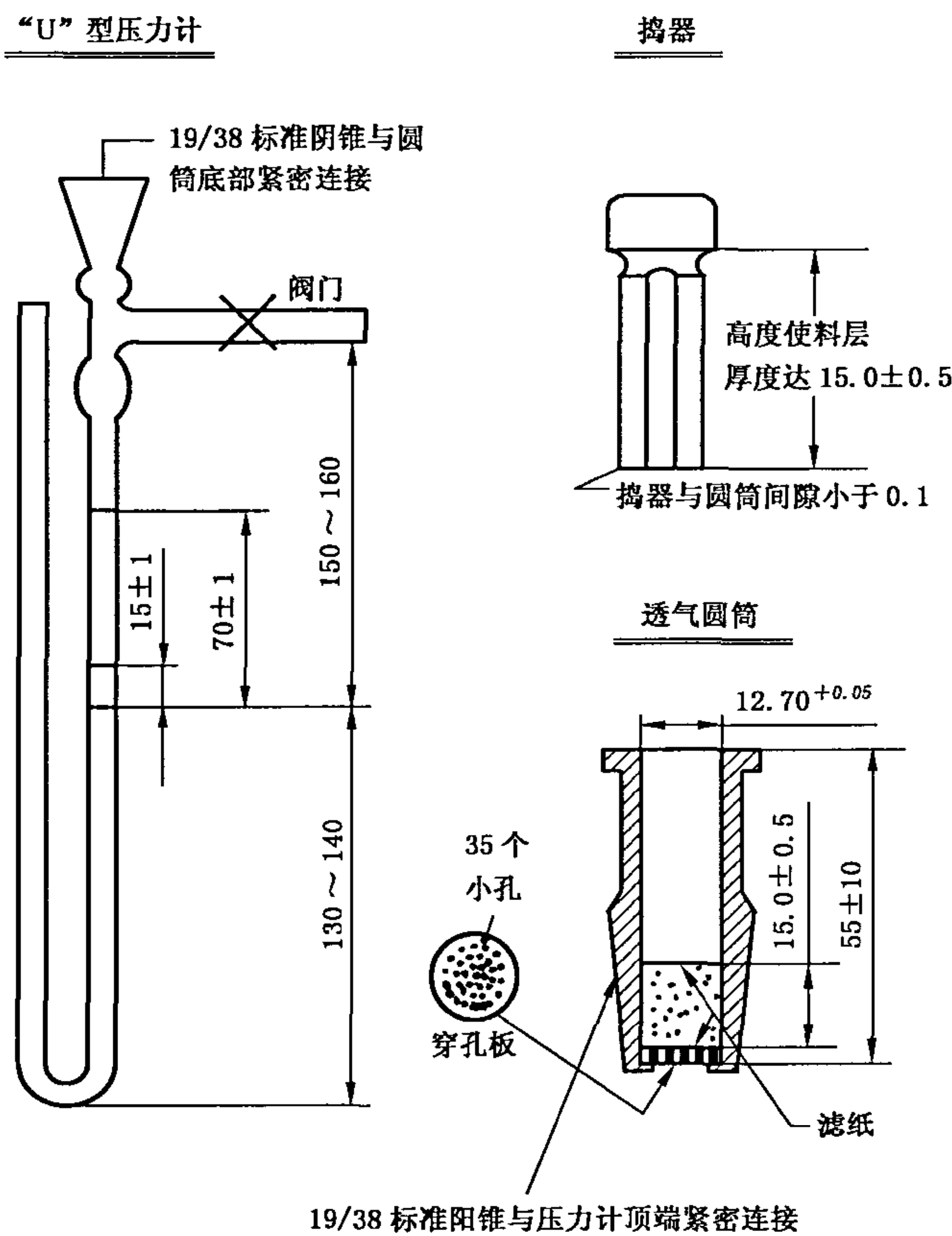
图 1 比表面积 U 型压力计示意图
