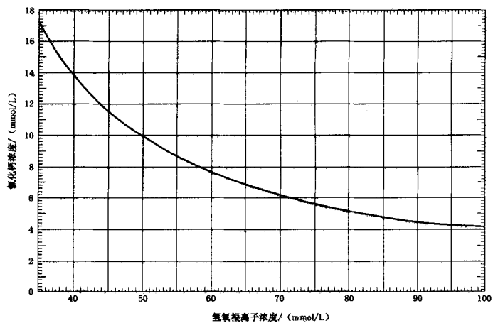
图 A.1 评定火山灰性的曲线图
